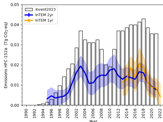
(d) HFC-152a
