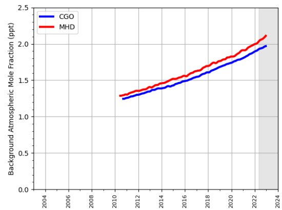
(d) PFC-318
