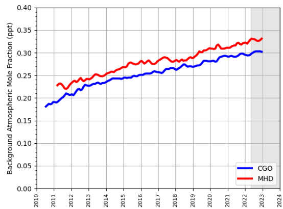
(d) HFC-43-10-mee
