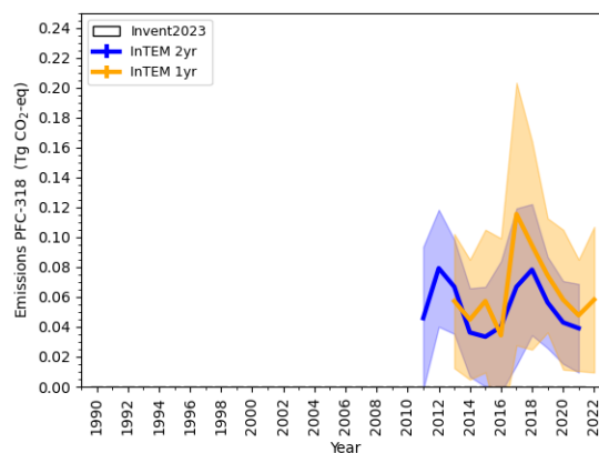
(d) PFC-318
