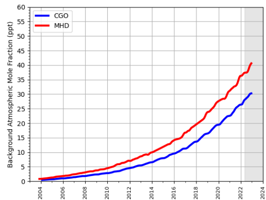
(d) HFC-32
