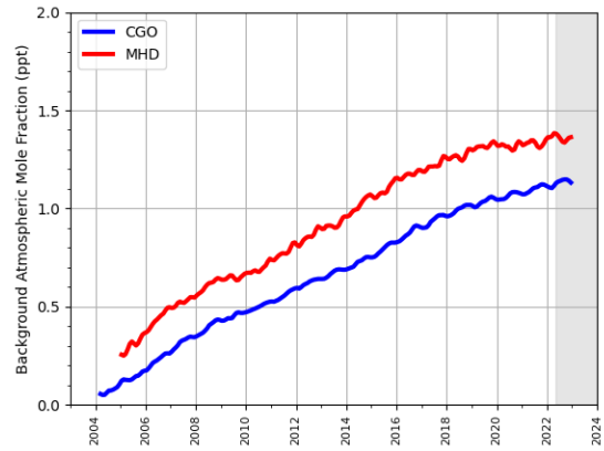
(b) HFC-365mfc
